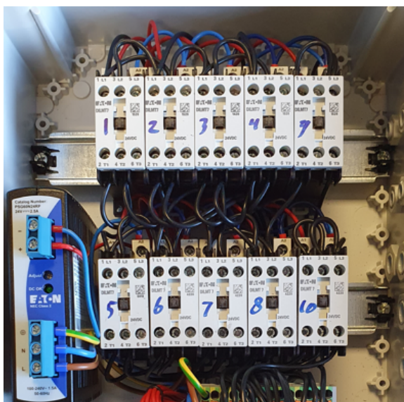
Figuur 3: nummering relais.
