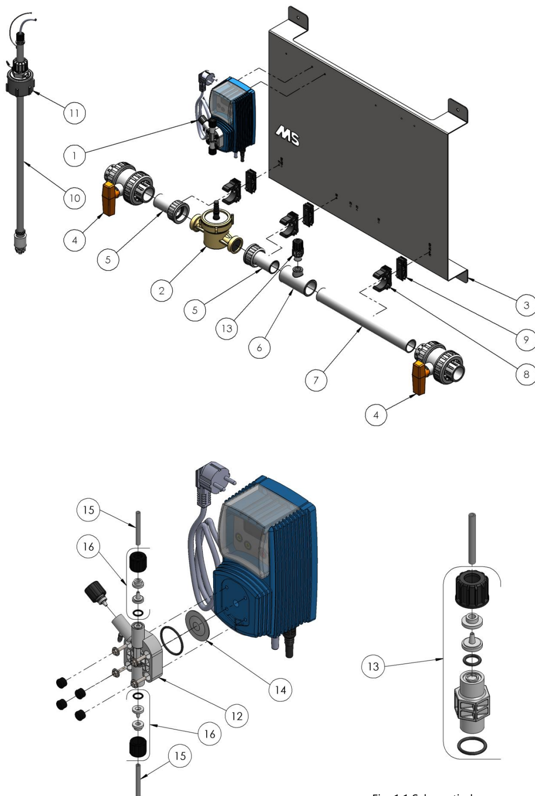
Fig. 1.1 Schematische weergave
