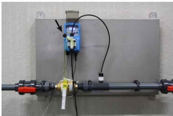
Afbeelding 11: Pomp ontluchten
