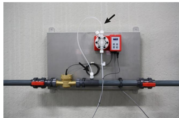
Afbeelding 4: Aansluiten persslang
