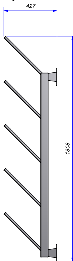
Zijaanzicht
